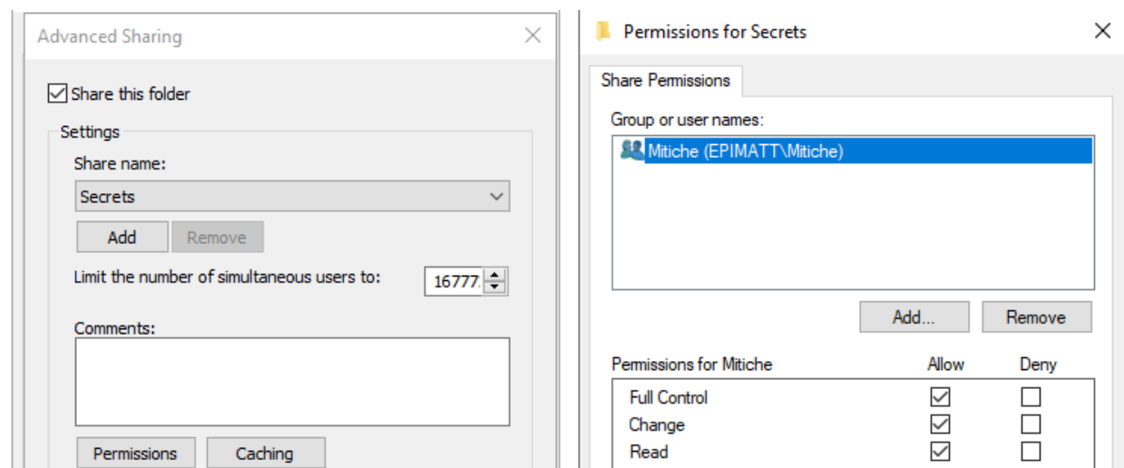
Figura 3: Configurazione delle "Share Permissions" per la cartella Secrets, assegnate al gruppo EPIMATT\Mitiche.
